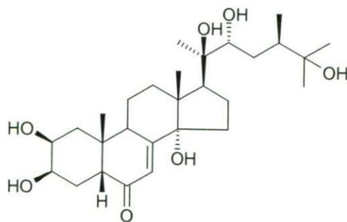
makisterone A (8)
