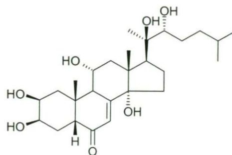
ajugasterone C (10)
