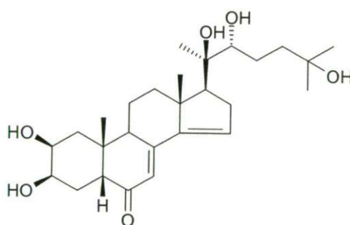
stachysterone B (6)
