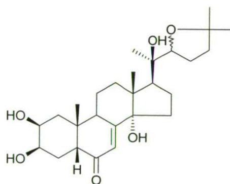
shidasterone (13)
