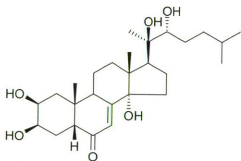
ponasterone A (5)
