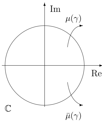
Neimark-Sacker bifurkáció
