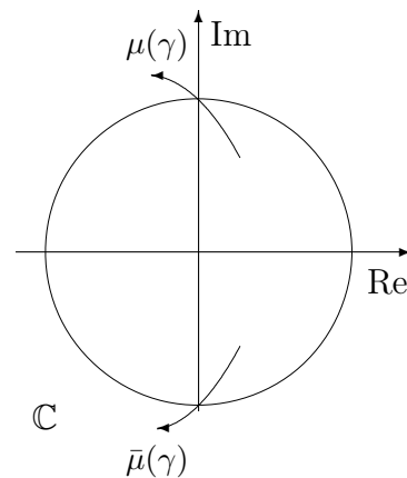
1:4 erős rezonancia
