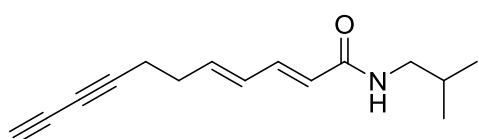
undeca-2 E ,4 E -diene-8,10-diynoic acid isobutylamide ( H. longipes )
