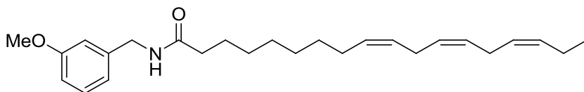
N -(3-methoxybenzyl)-9 Z ,12 Z ,15 Z -octadecatrienamide
