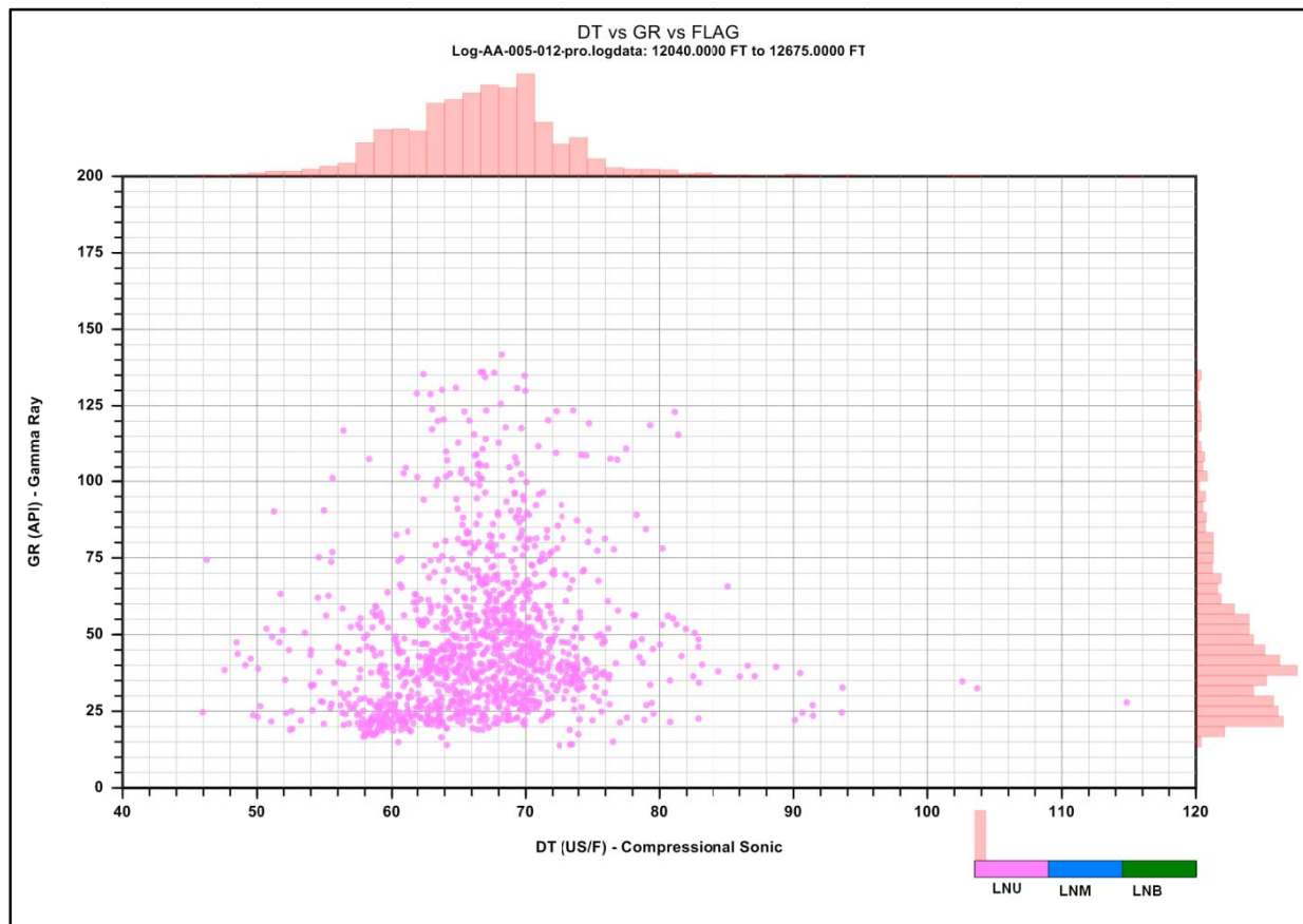
Fig. 1-16 Interpretation Parameters well: 2A5
