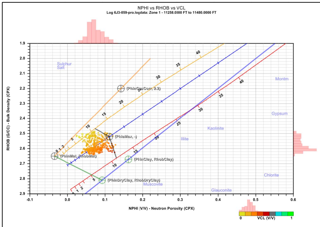
Fig. 1-4 Interpretation Parameters well: 6J3
