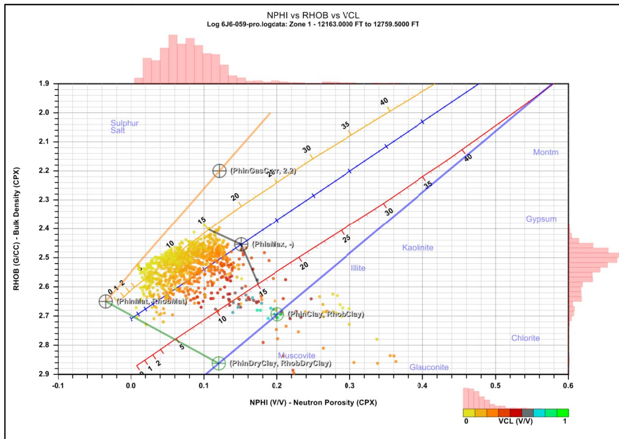
Fig. 1-6 Interpretation Parameters well: 6J6
