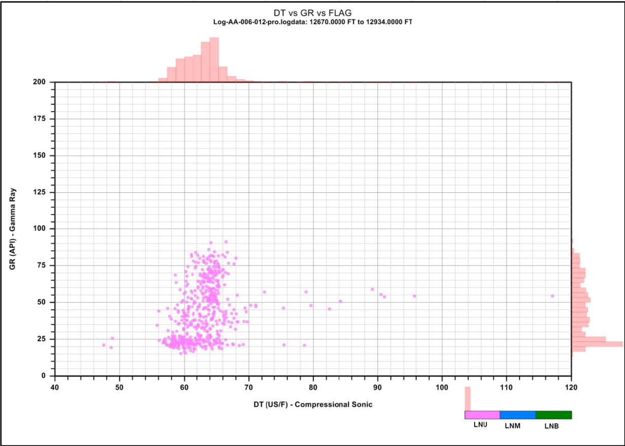
Fig. 1-17 Interpretation Parameters well: 2A6
