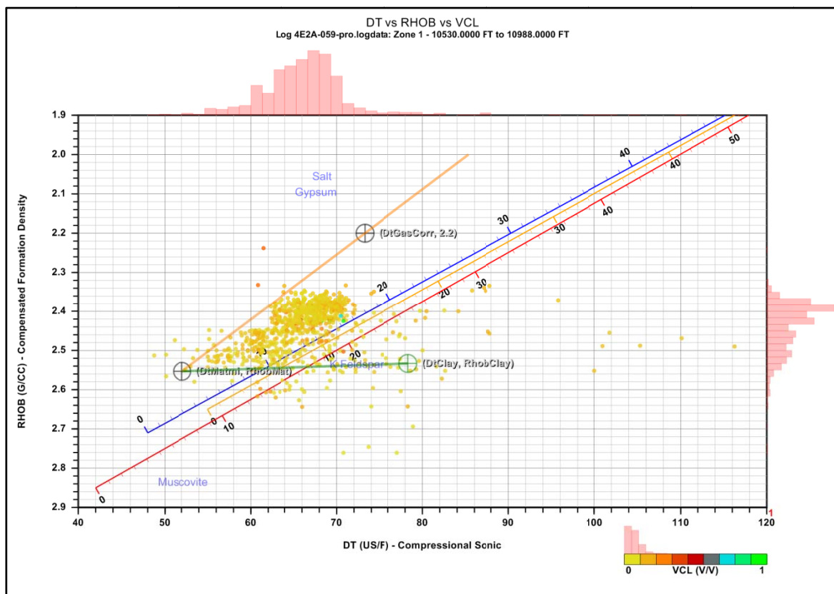
Fig. 1-2 Interpretation Parameters well: 4E2A
