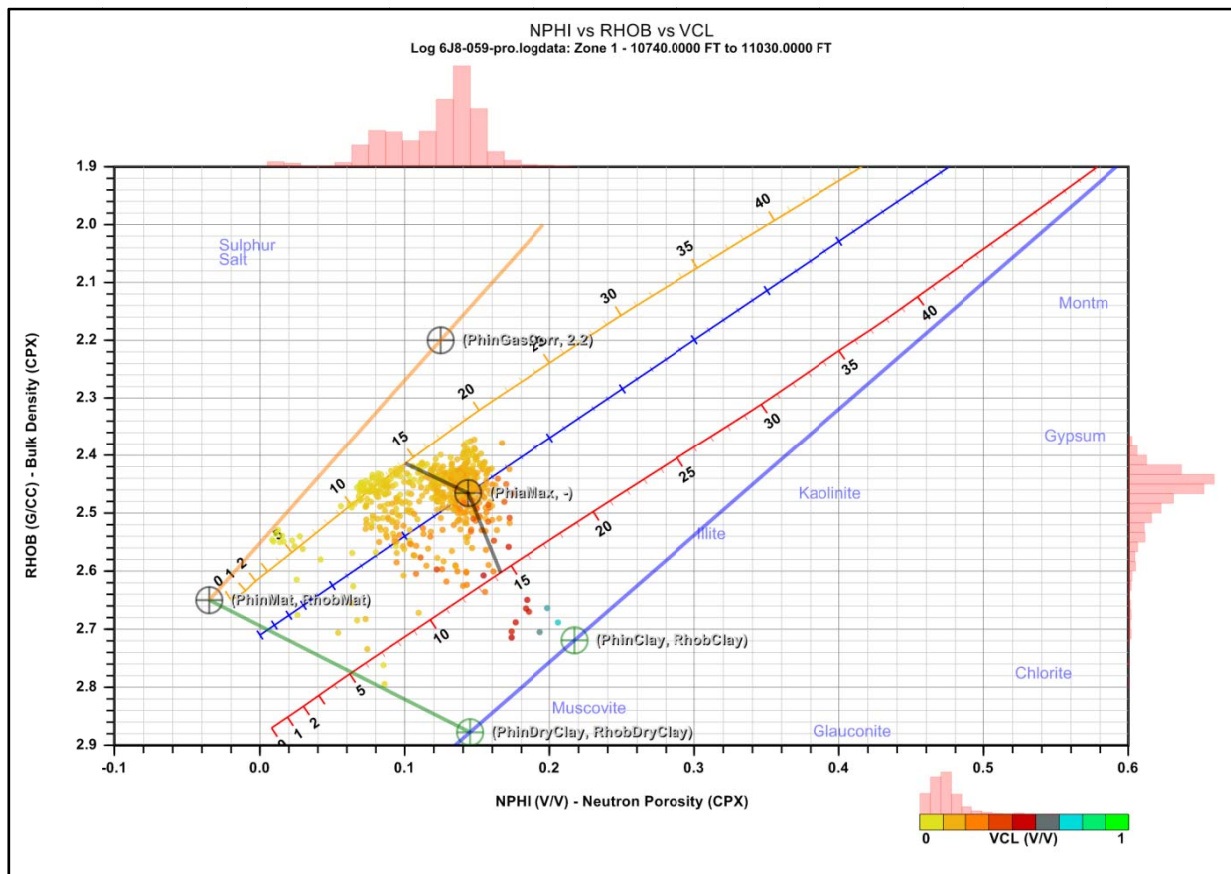
Fig. 1-8 Interpretation Parameters well: 6J8
