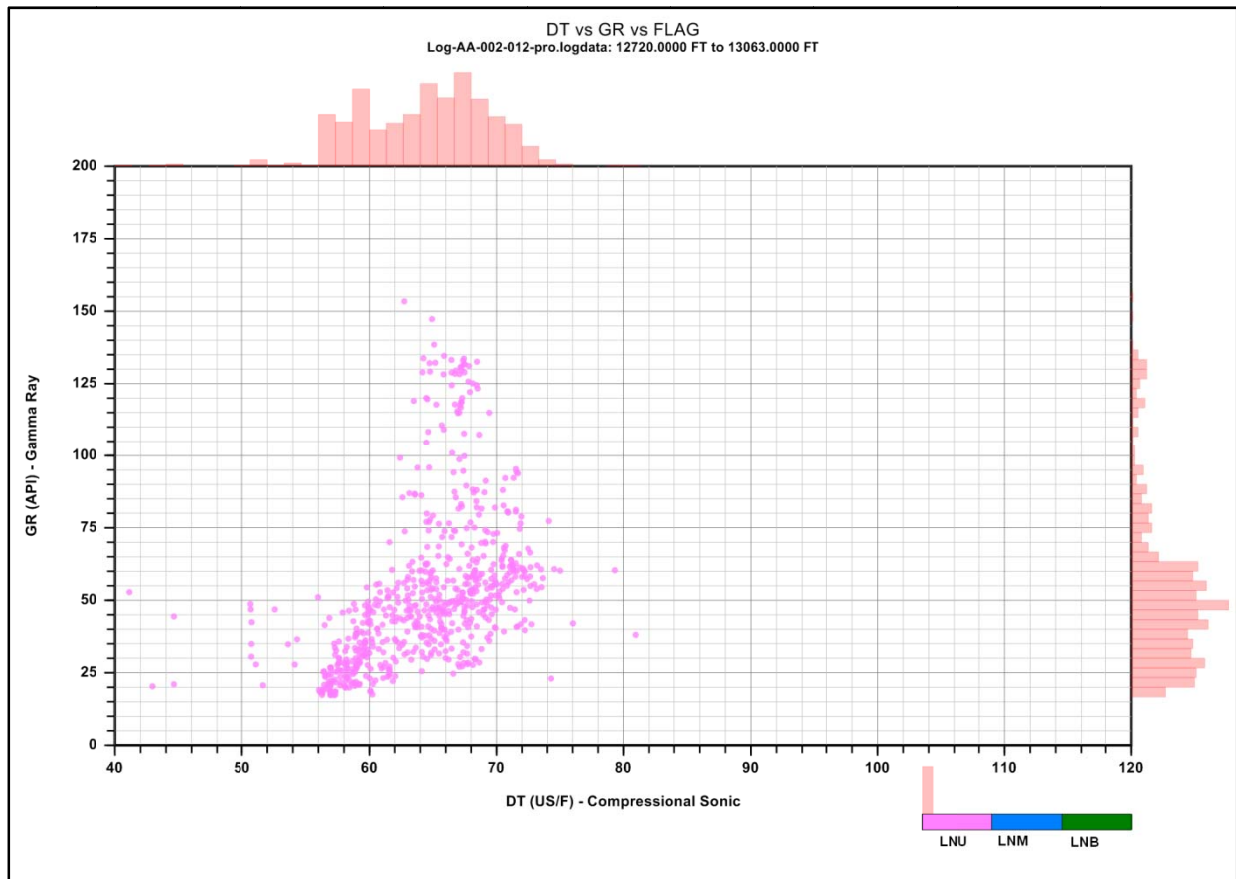
Fig. 1-13 Interpretation Parameters well: 2A2
