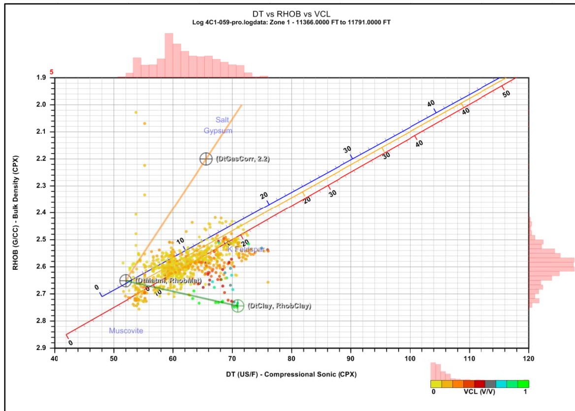
Fig. 1-1 Interpretation Parameters well: 4C1
