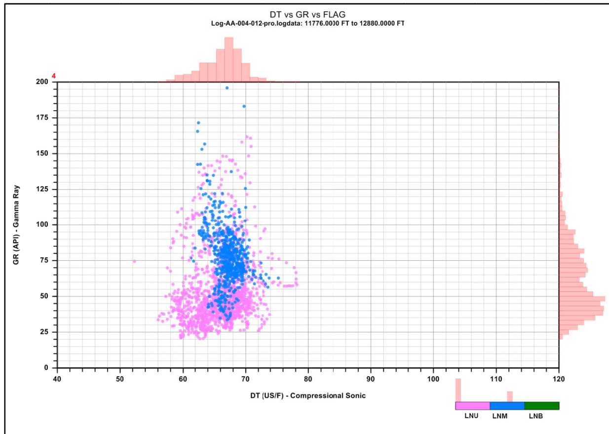
Fig. 1-15 Interpretation Parameters well: 2A4
