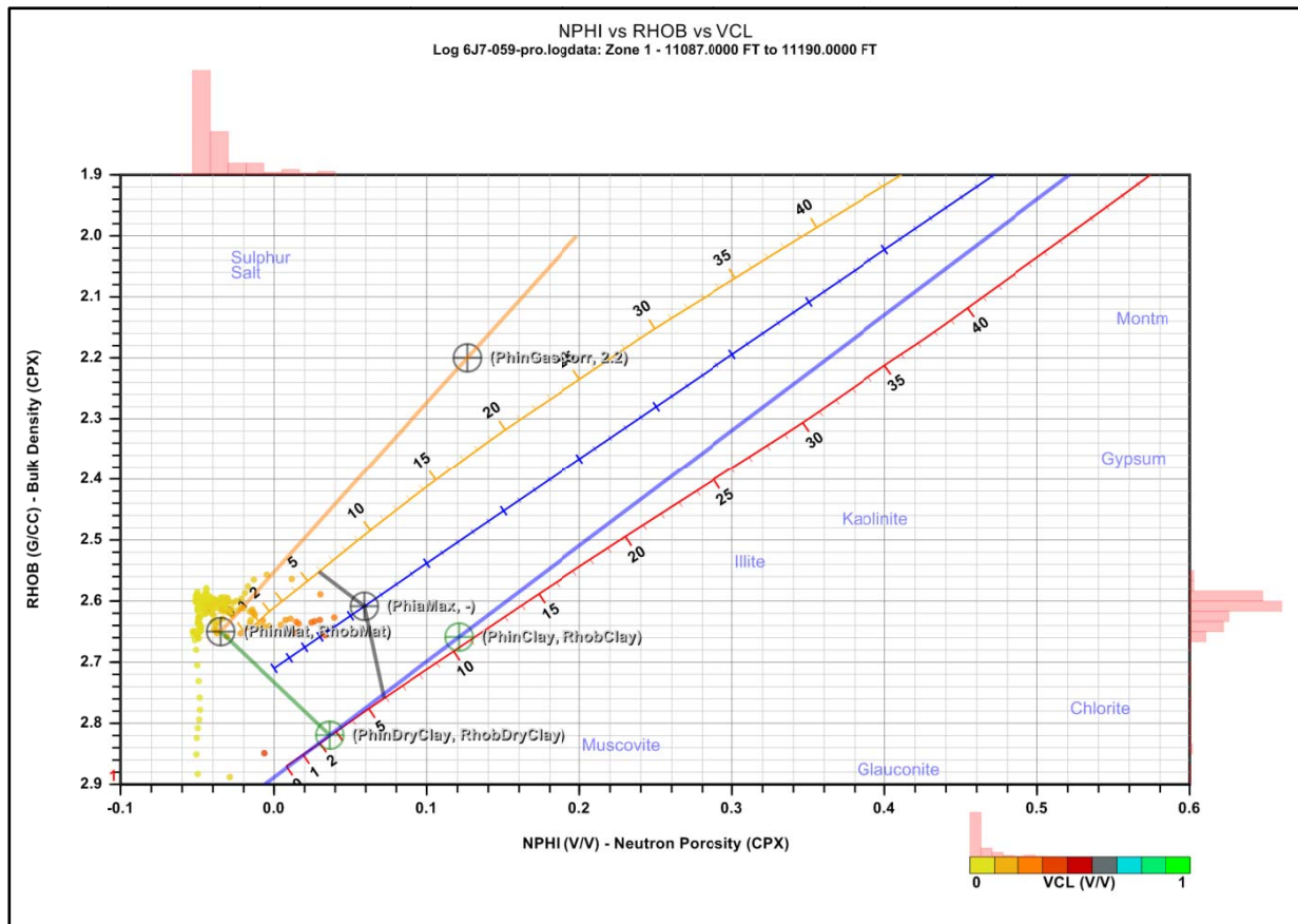
Fig. 1-7 Interpretation Parameters well: 6J7
