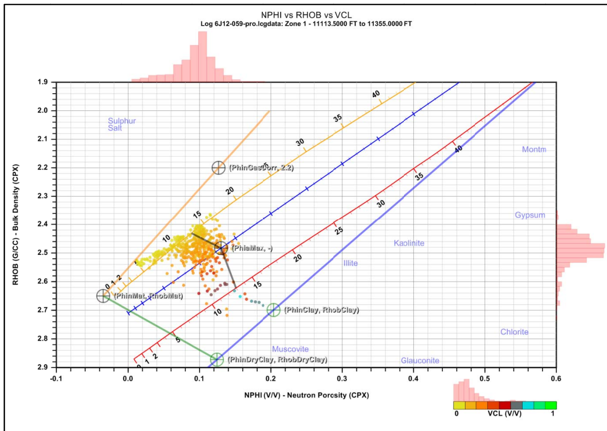
Fig. 1-10 Interpretation Parameters well: 6J12
