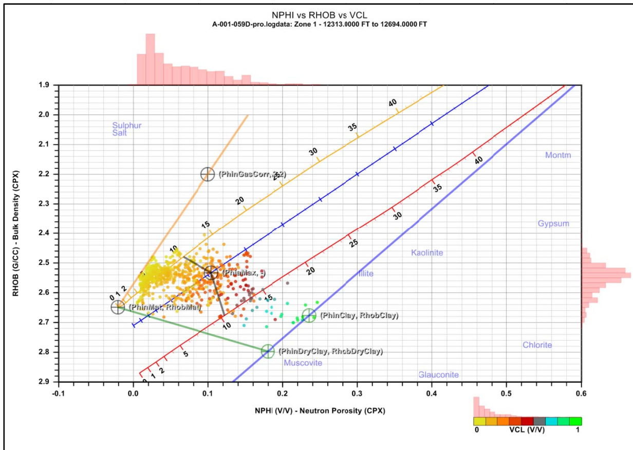
Fig. 1-11 Interpretation Parameters well: A1
