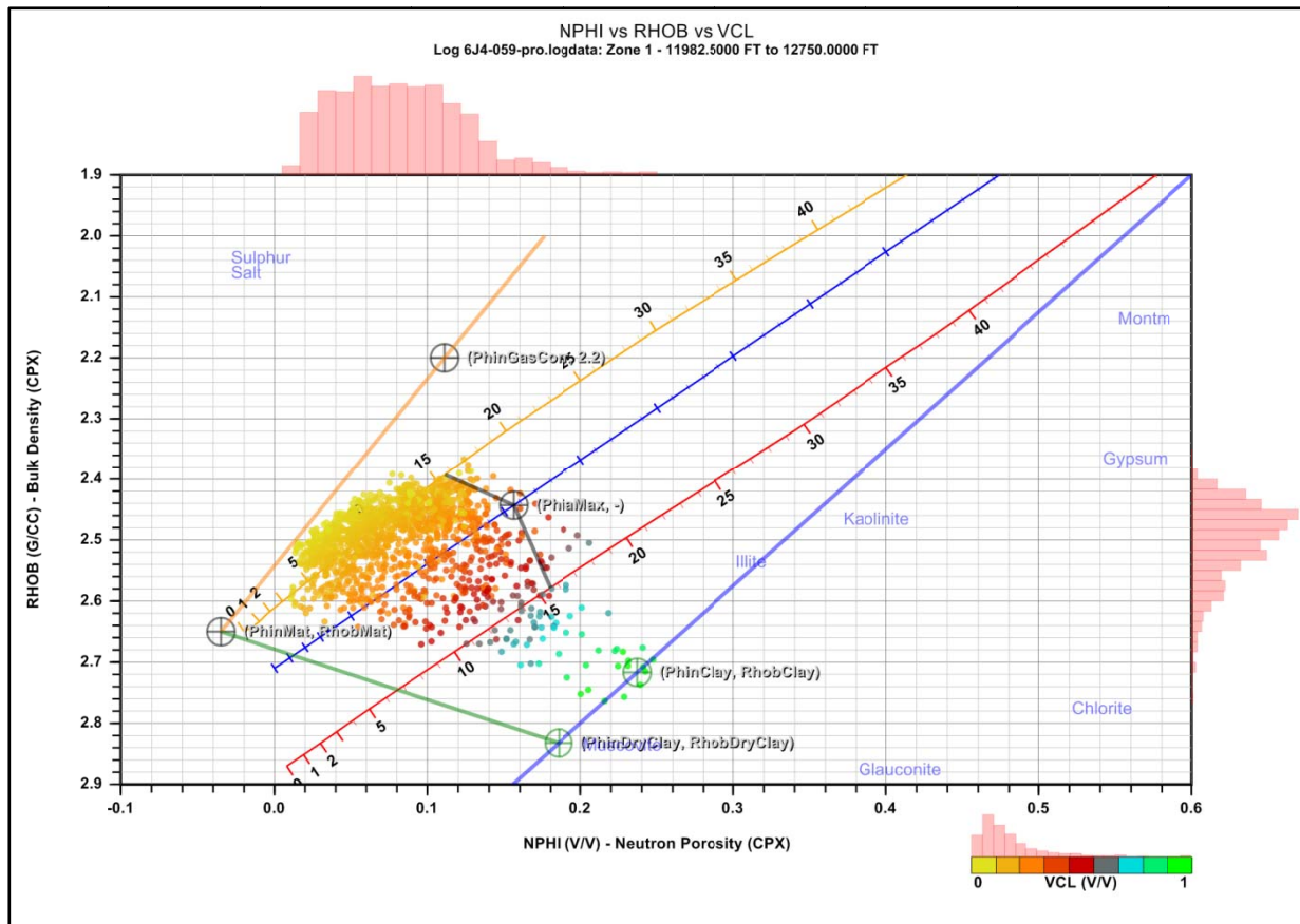
Fig. 1-5 Interpretation Parameters well: 6J4
