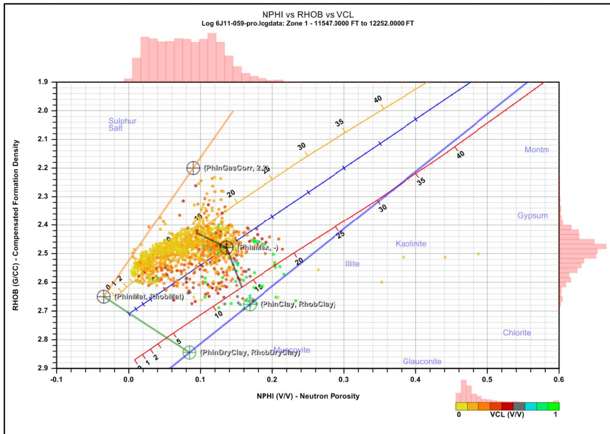
Fig. 1-9 Interpretation Parameters well: 6J11
