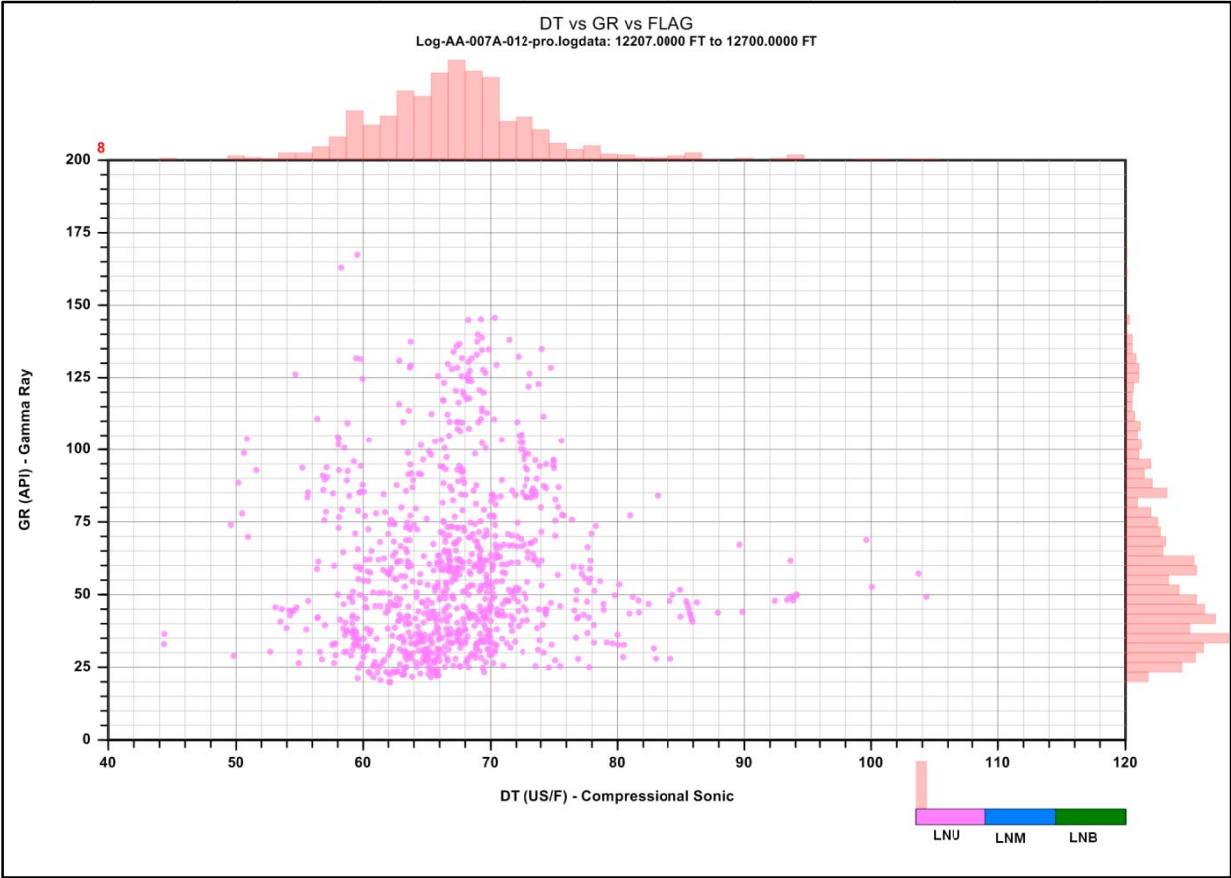
Fig. 1-18 Interpretation Parameters well: 2A7A
