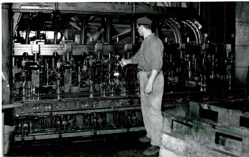
2. kép. Korszerű öblösüveggyártó automatagép
