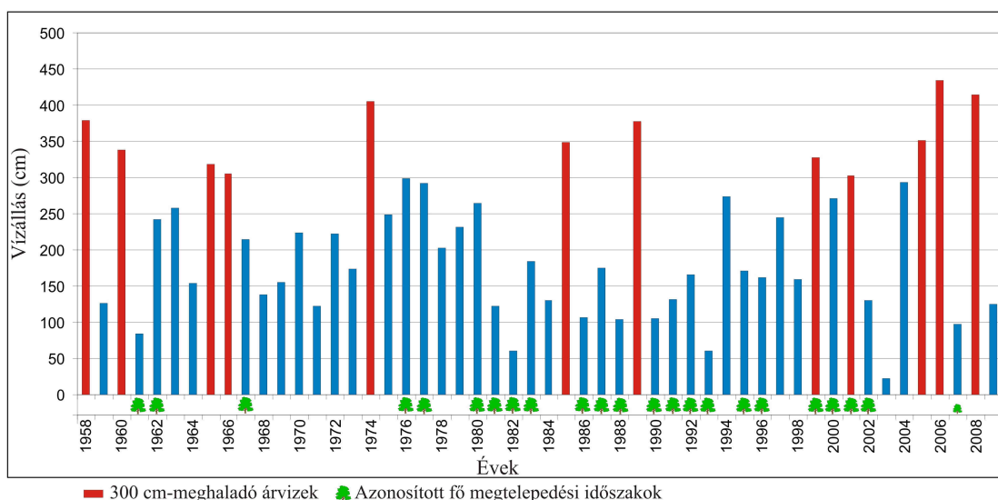
4.37. ábra: Az évi legnagyobb vízállások a dendrológiai vizsgálat időszakában (Hidasnémeti vízmérce alapján), valamint a kiemelkedően nagy árvizek és a főbb megtelepedési időszakok.
