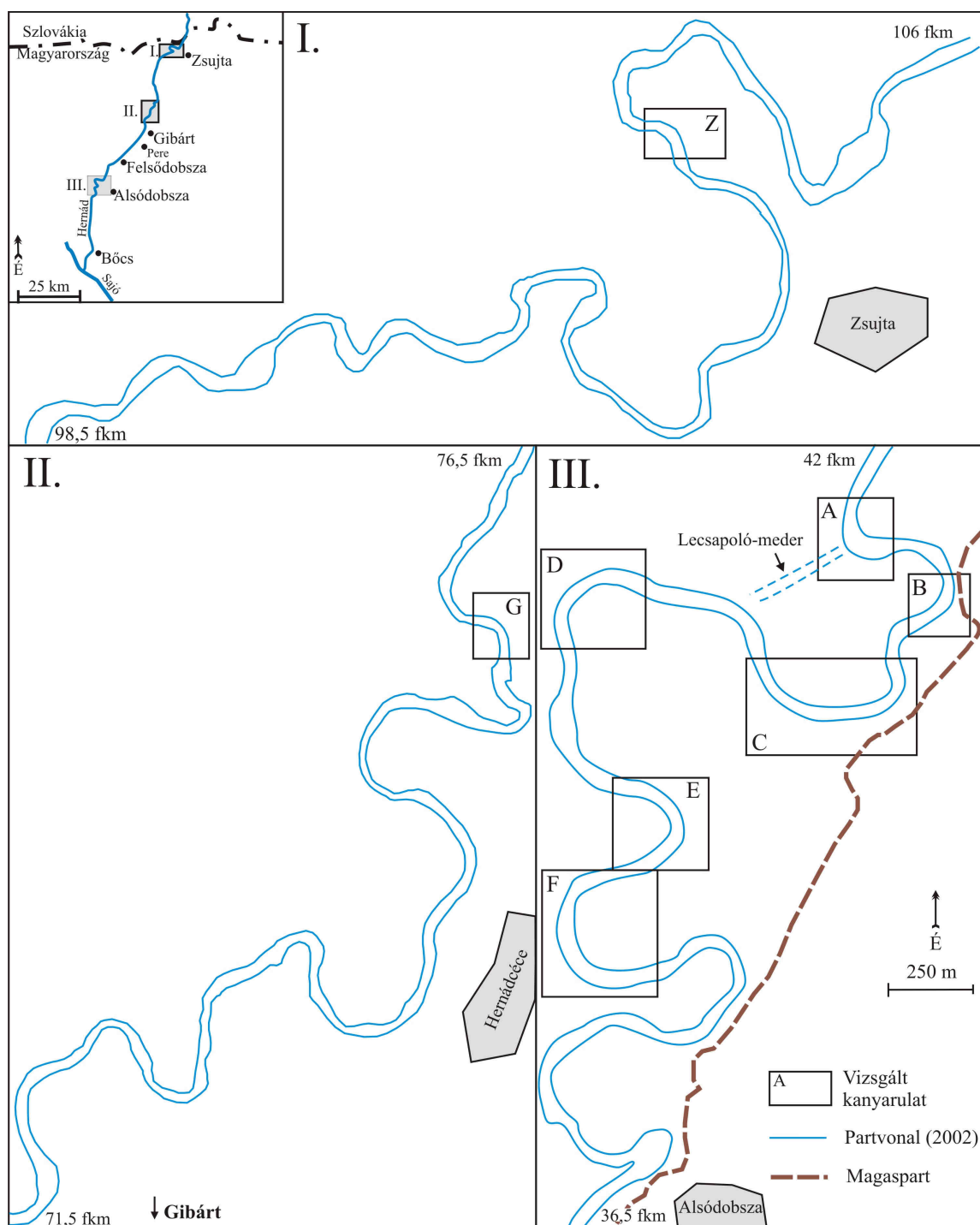
4.25. ábra: A vizsgált kanyarulatok elhelyezkedése a zsujtai (I.), a gibárti (II.) és az alsódobszai (III.) szakaszokon
