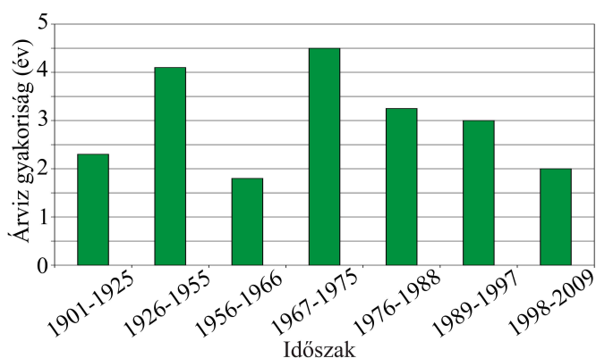
4.7. ábra: Az árvizes évek gyakorisága az időszakokon belül az egyes időszakokban
