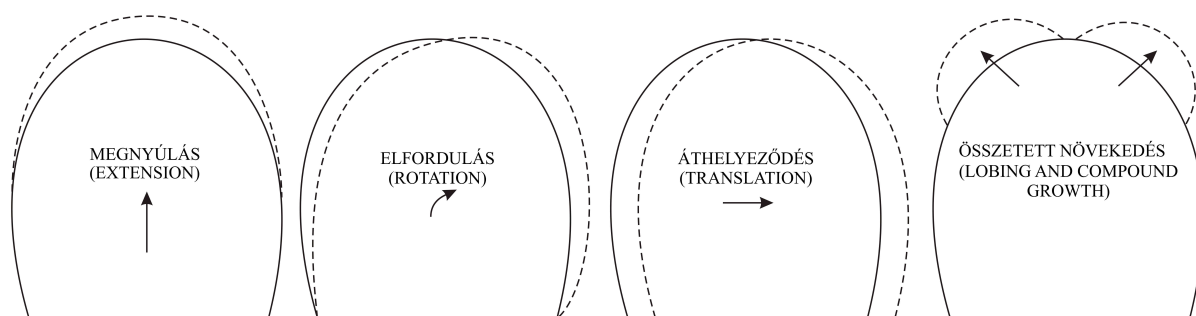
1.6. ábra: A kanyarulatfejlődés típusai Nanson és Hickin (1983) alapján
