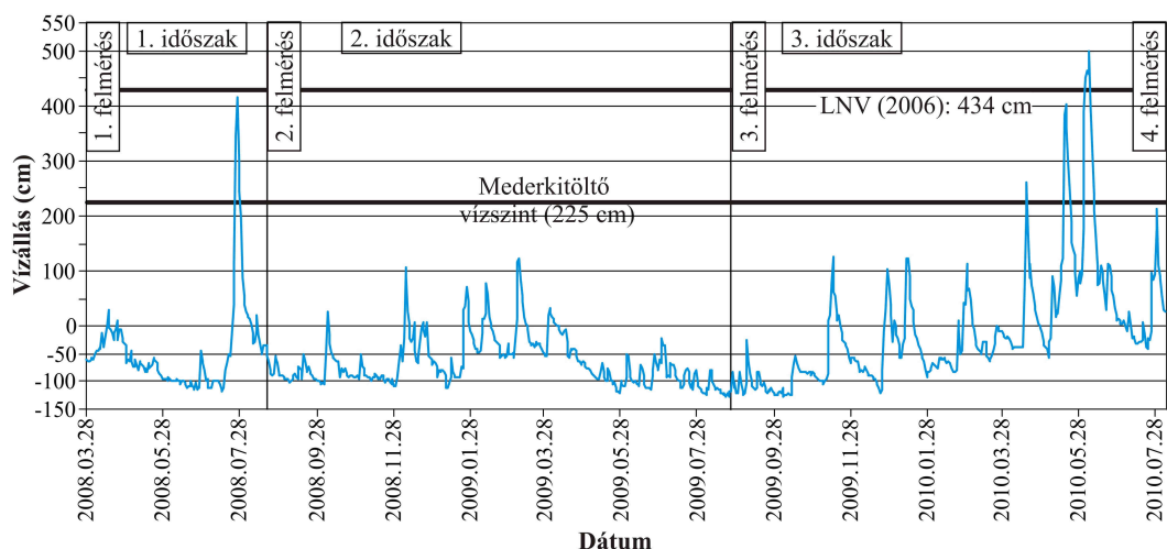
4.28. ábra: A vizsgált időszak (2008.03.28.-2010.08.06.) vízjárása a hiasnémeti vízmérce alapján
