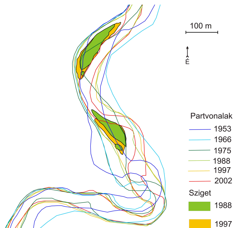
4.16. ábra: A partvonal futásának változása 1953-2002 között a gíbárti szakaszon
