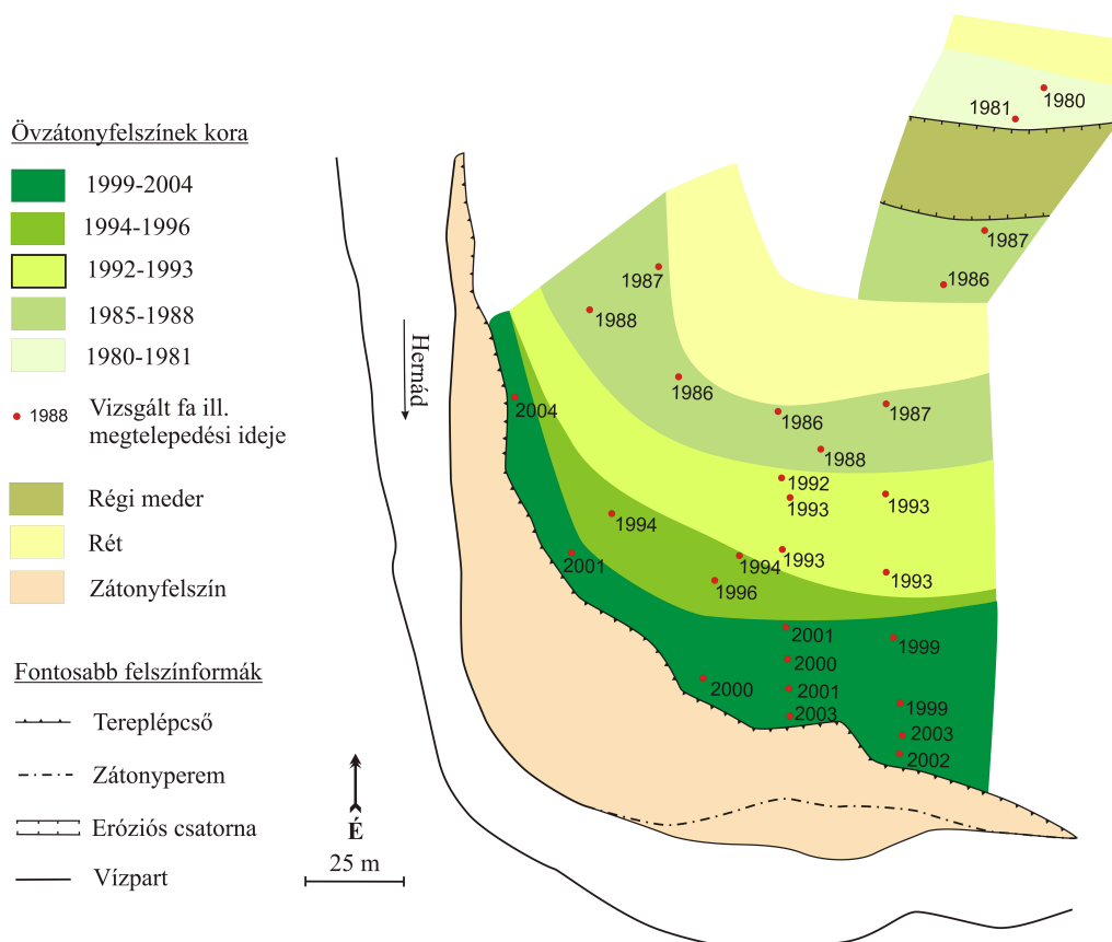
4.38. ábra: A fák kora alapján meghatározott övzátony-épülési periódusok az alsódobszai A kanyarulatban
