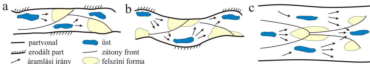
1.2. ábra: A gázlók és üstök mintázata egyenes a), meanderező b) és fonatos mederben c) (Ferguson 1993)
