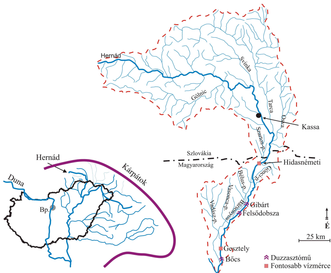
2.1. ábra: A Hernád vízgyűjtője
