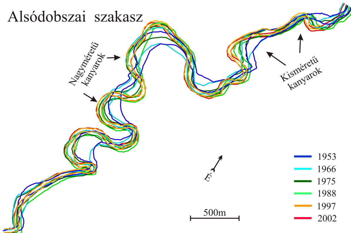
4.15 b. ábra: A partvonal futásának változása és a kis- és nagyméretű kanyarulatok elhelyezkedése az alsódobszai szakaszon 1953-2002 között
