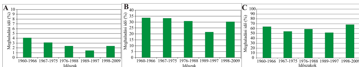
4.5. ábra: a) a mederformáló vízhozamot b) a közép-vízhozamot és c) a kisvizet meghaladó vízhozamok időtartama az össz-időtartam %-ában
