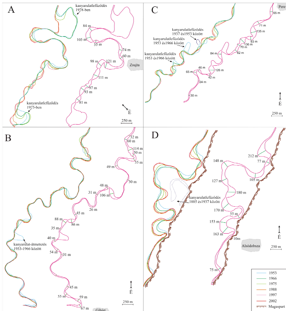
4.13. ábra: A) A középvonal helyzete az egyes időpontokban 1953 és 2002 között és a teljes középvonal elmozdulás 1953 és 2002 között zsujtai (A), gibárti (B), a pereji (C) és az alsódobszai szakaszon (D).
