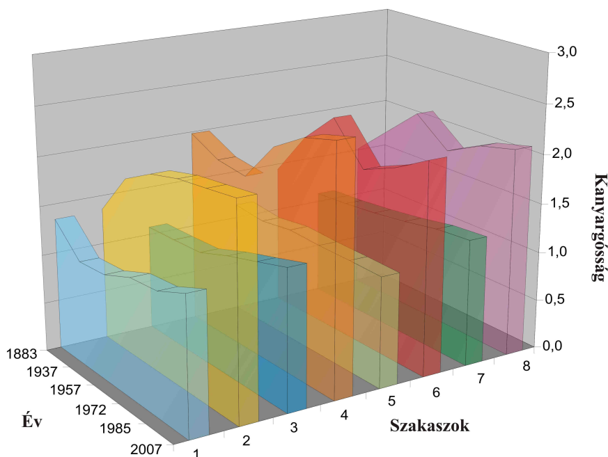
4.18. ábra: A kanyargósság változása az egyes szakaszokon
