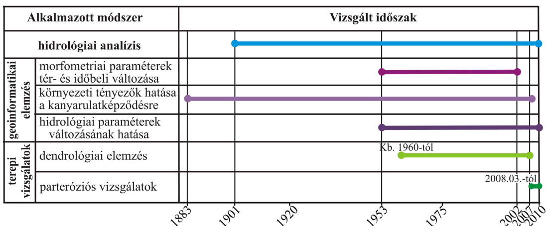
3.2. ábra: A különböző vizsgálatok által felölelt időszakok
