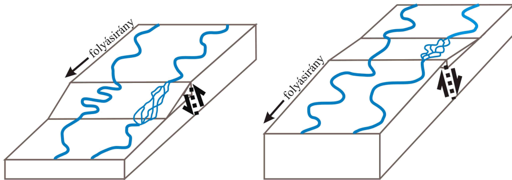
1.8. ábra: Meanderező folyó kanyarfejltségének és alaktípusának változása a meder merőleges vető hatására a) a völgylejtés növekedése és b) csökkenése következtében ( Tímár 2005)
