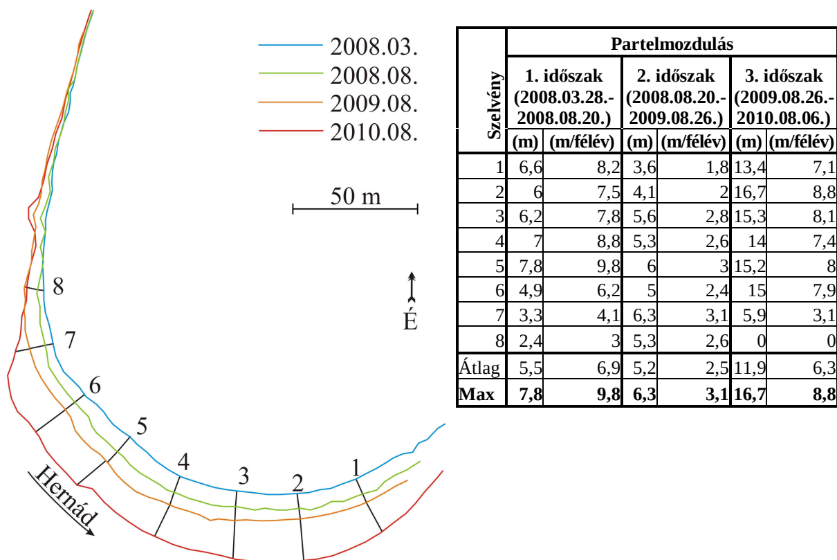
4.26. ábra: Rövid távú partelmozdulás az alsódobszai A kanyarulat külső ívén 2008-2010. között és az elmozdulás jellemző abszolút értéke és félèves üteme
