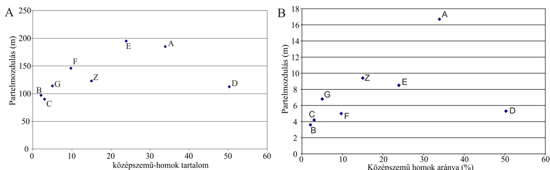
4.33. ábra: A partanyag középszemű-homok tartalma és a partelmozdulás kapcsolata az 1953-2007 közötti a) , valamint a 2009.08.-2010.08. közötti b) időszakban
