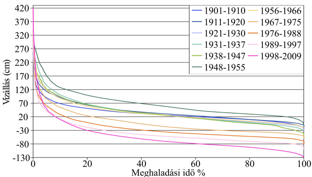
4.3. ábra: A vízállástartósságok (1901-2009) az egyes időszakokban
