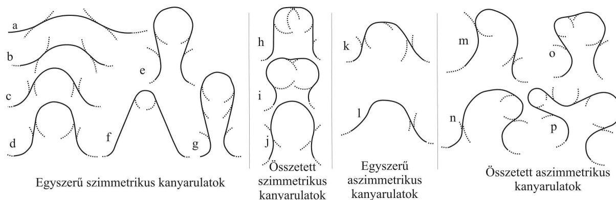
1.9. ábra: Kanyarulat mintázatok (Brice 1974)
