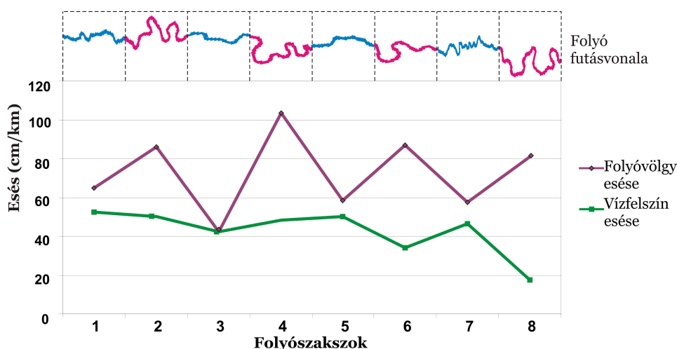
4.19. ábra: A vízfelszín átlagos esése az egyes szakaszokon és a völgyszakaszok átlagos esése a vizsgált folyószakaszon
