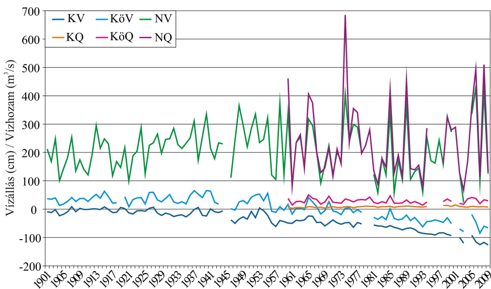
4.6. ábra: Évi legnagyobb, legkisebb és közepes vízállások (1901-2009) és vízhozamok (1960 -2009) alakulása
