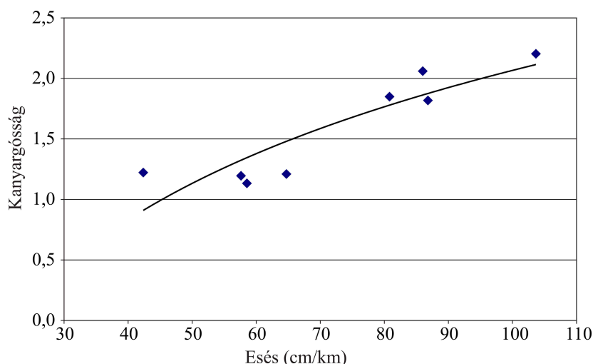
4.20. ábra: Az esés és a kanyargósság kapcsolata a vizsgált folyószakaszon
