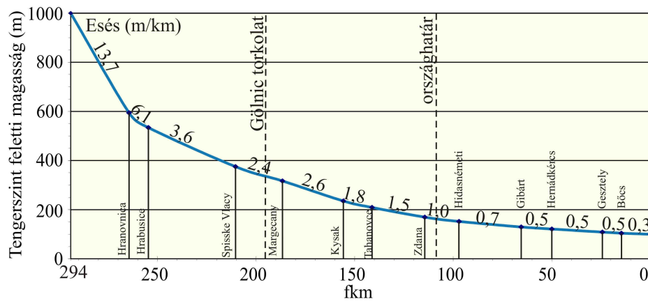
2.2. ábra: A Hernád esésgörbéje a vízmércék 0 pontjai alapján (saját számítások alapján)
