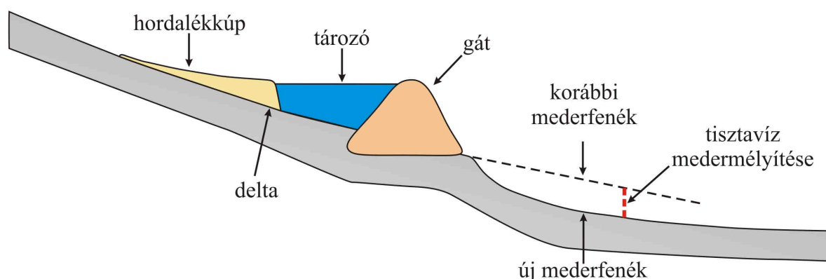
1.11.ábra: A duzzasztók hatása az alvizi és a felvizi irányában (Szabó 2006)
