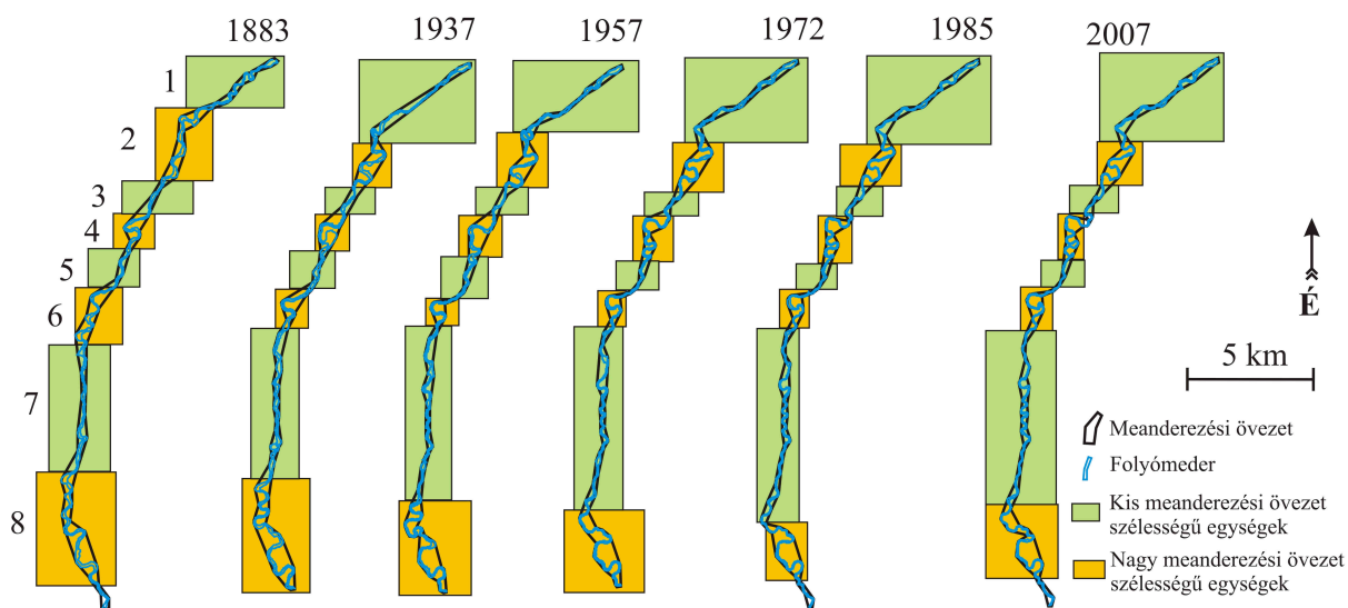
4.17. ábra: A meanderezési övezet szélessége és az eltérő kanyargósságú egységek 1883 és 2007 között a Felsődobsza Bőcs közötti folyószakaszon
