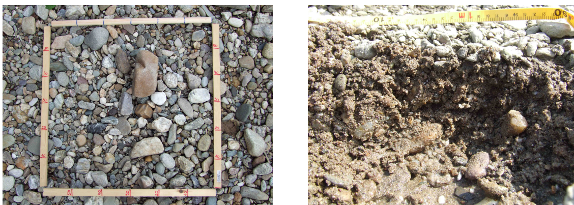
2.9. ábra: Mederanyag az övzátonyokon Hidasnémeti felett és Alsódobsza közelében
