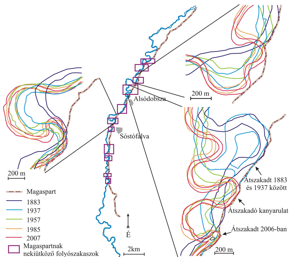
4.24. ábra: Kanyarulatfejlődés a magaspartnak nekiütköző folyószakaszokon
