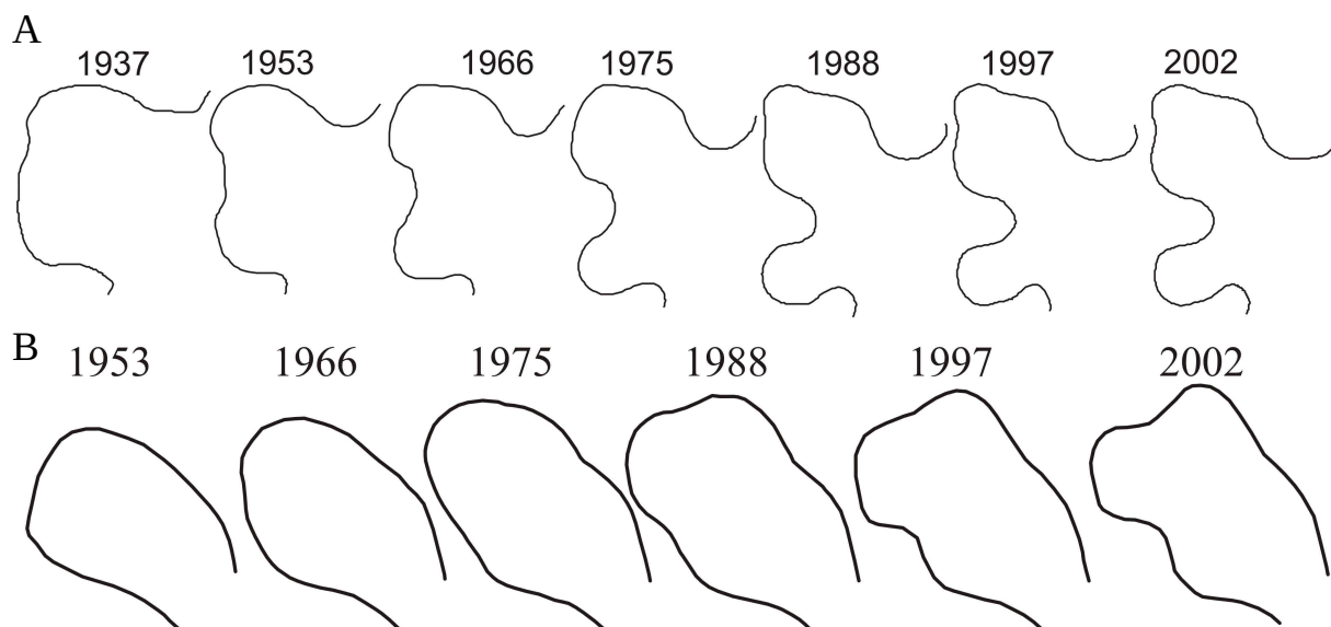
4.14. ábra: Összetett kanyarulat fejlődése Alsódobszánál A) és Zsujtánál B)
