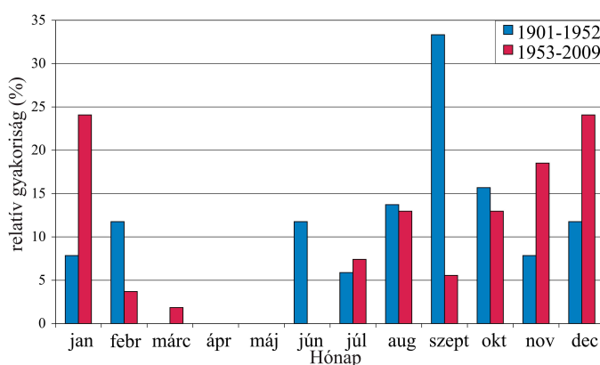
4.11. ábra: Az évi legkisebb napi vízállások relatív gyakorisága az egyes hónapokban 1953 előtt és után a Hidasnémeti vízmércénél
