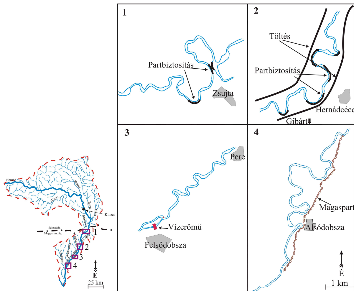
2.10. ábra: A mintaterületek elhelyezkedése
