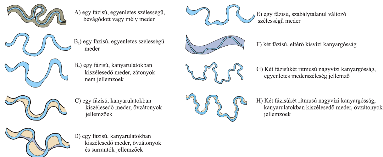
1.10. ábra: Brice (1974) osztályozási rendszerének módosított változata (Hooke 2007b).
