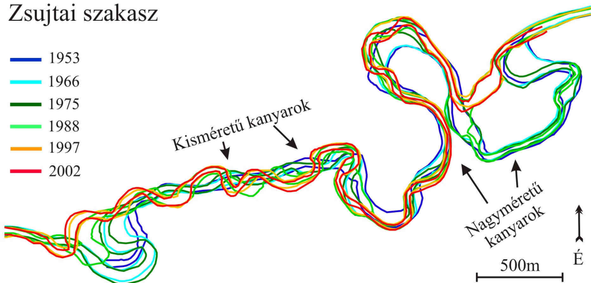
4.15 a. ábra: A partvonal futásának változása és a kis- és nagyméretű kanyarulatok elhelyezkedése a zsujtai szakaszon 1953-2002 között
