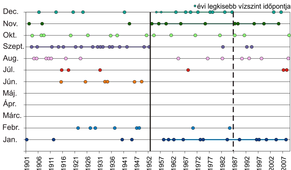
4.10. ábra: Az évi legkisebb vízállások hónapokénti megoszlása a Hidasnémeti vízmércénél
