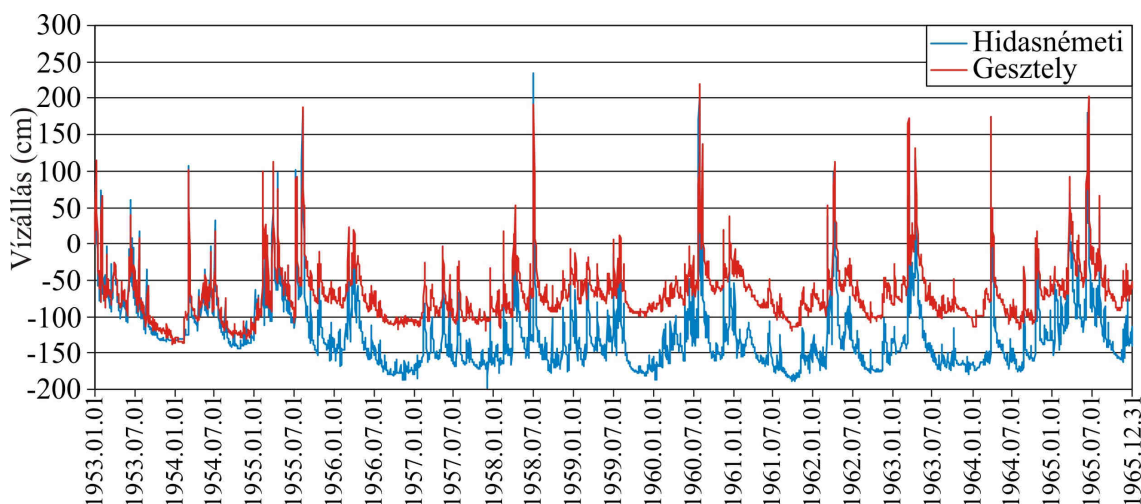
4.2. ábra: Vízállás a hidasnémeti és a gesztelyi vízmércén 1953-1965 között
