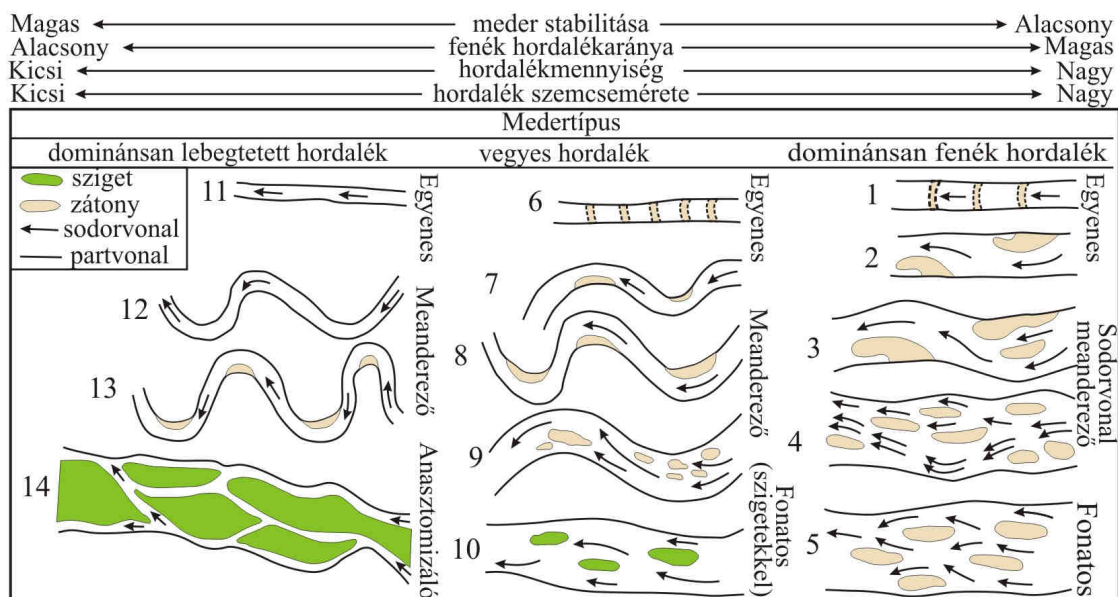
1.1. ábra: Alluviális medrek mintázat típusai (Schumm 1985 alapján)
