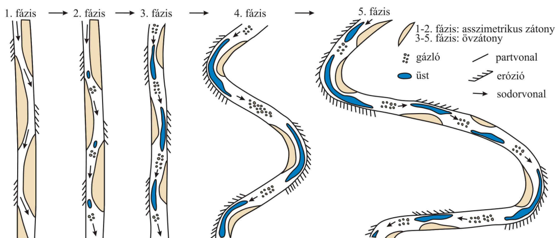
1.5. ábra: A meanderezés kialakulása és fejlődése (Keller 1972)
