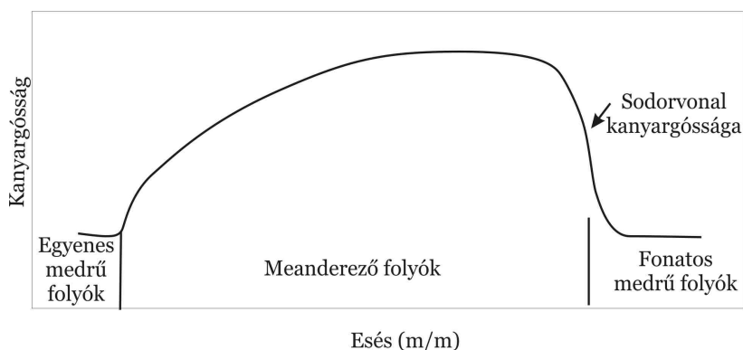
1.3. ábra: Az esés és a kanyargósság kapcsolata (Schumm és Khan 1972)
