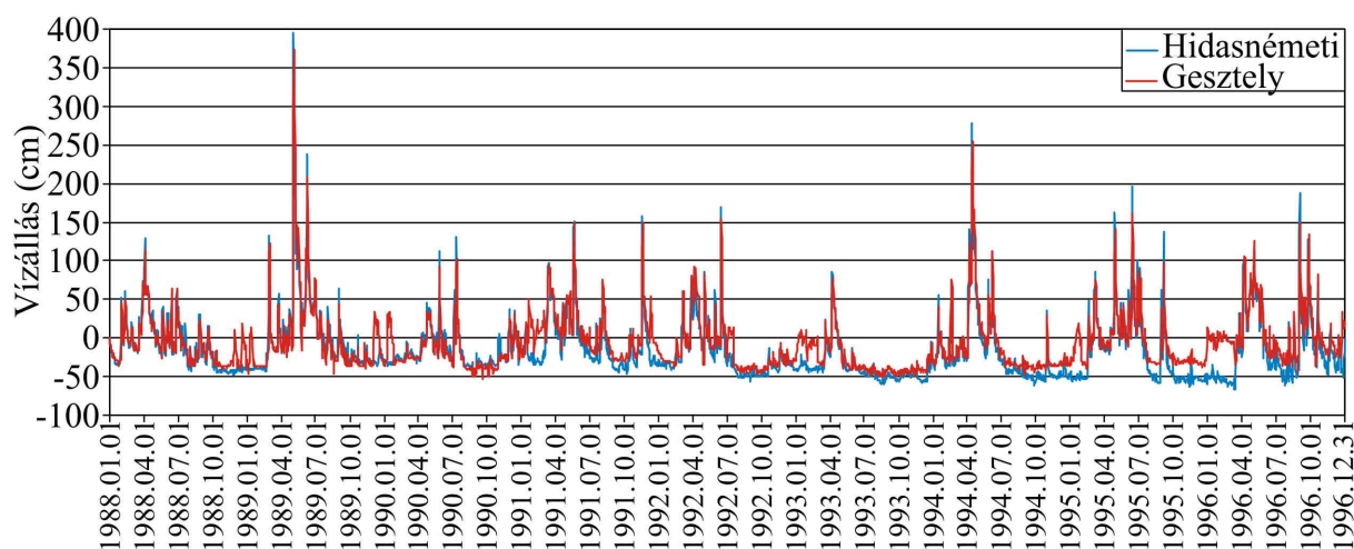
4.1. ábra: A kezdő időponthoz (1988.01.01) viszonyított vízállás a hidasnémeti és a gesztelyi vízmércén 1988-1996 között
