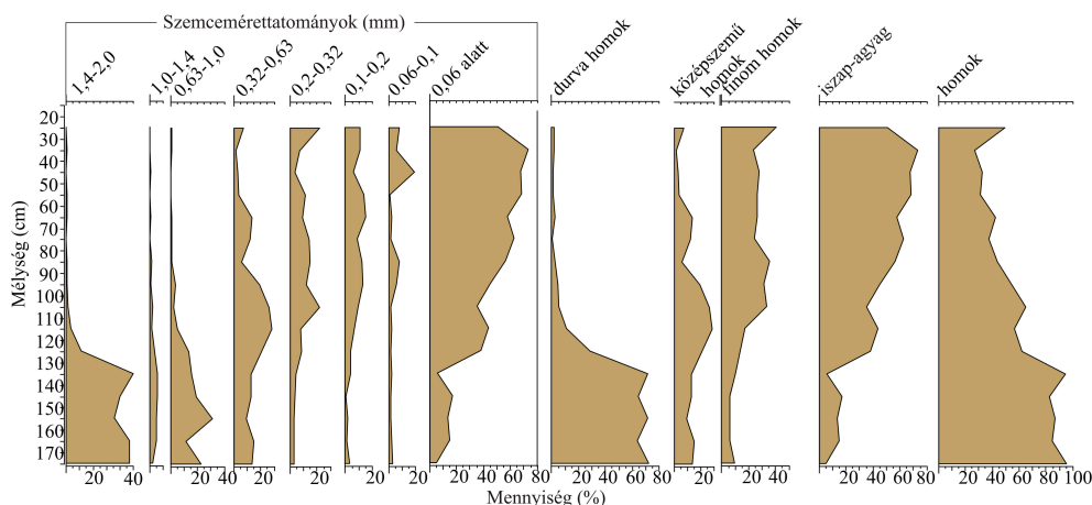
4.30. ábra: A szemcseösszetétel változása a zsujtai Z kanyarulat fúrásszelvényében
