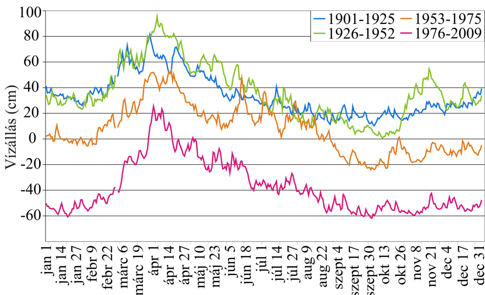
4.9. ábra: A vízállásértékek napi átlagértékei az 1901-1925, 1926-1952, 1953-1975 és 1976-2009 időszakokra lebontva a Hidasnémeti vízmércénél.
