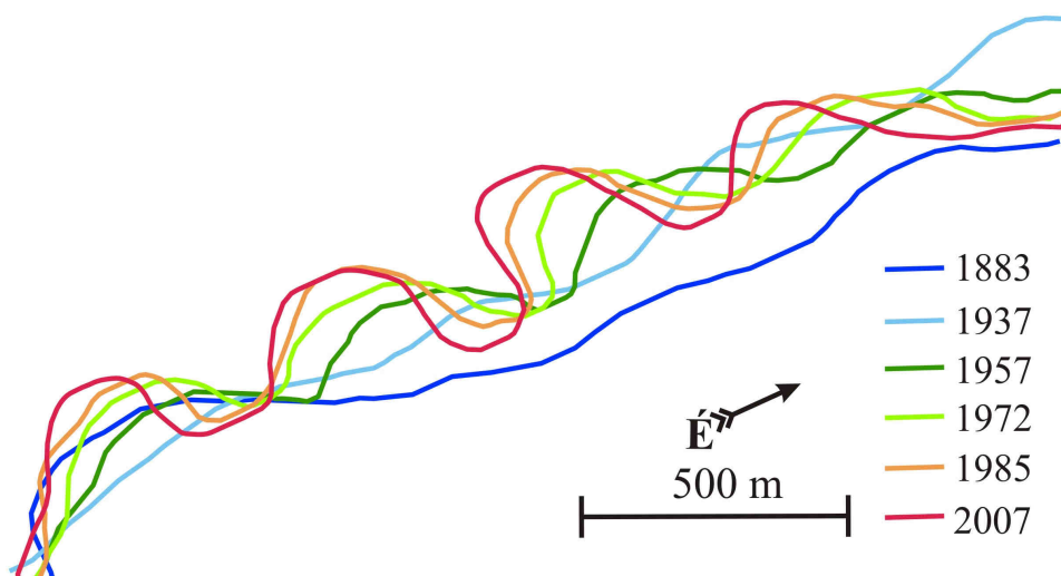
4.21. ábra: A középvonal helyzete a gyengén kanyargós (7.) egységen 1883 és 2007 között
