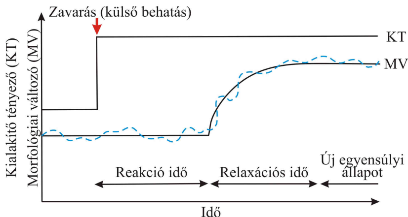
1.4.ábra: A rendszer reakció- és relaxációs ideje a rendszert ért zavarást követően (Brunsden 1980)
