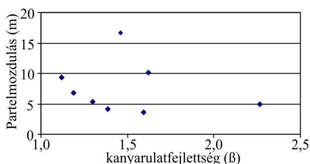
4.34. ábra: A kanyarulat-fejlettség és a 2009.08.-2010.08. közötti időszakban megfigyelhető partelmozdulás kapcsolata
