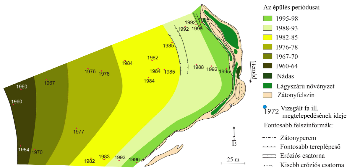
4.38. ábra: A fák kora alapján meghatározott övzátony-épülési periódusok az alsódobszai E kanyarulatban
