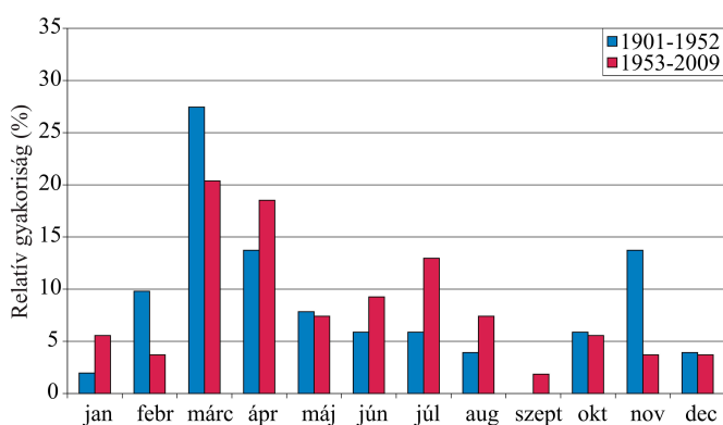
4.12. ábra. Az évi legnagyobb napi vízállások relatív gyakorisága az egyes hónapokban 1953 előtt és után a Hidasnémeti vízmércénél
