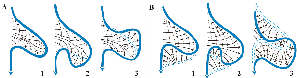
1.7.ábra: Az összetett kanyarulatok fejlődése, ha az inflexiós pontok helyben maradnak és a kanyarulat ívén egy másodlagos ív alakul ki A) és ha szomszédos kanyarulat felső oldala belefejlődik a kanyarulatba B). (a szaggatott vonal a partvonal korábbi futását mutatja) (Hickin 1974)
