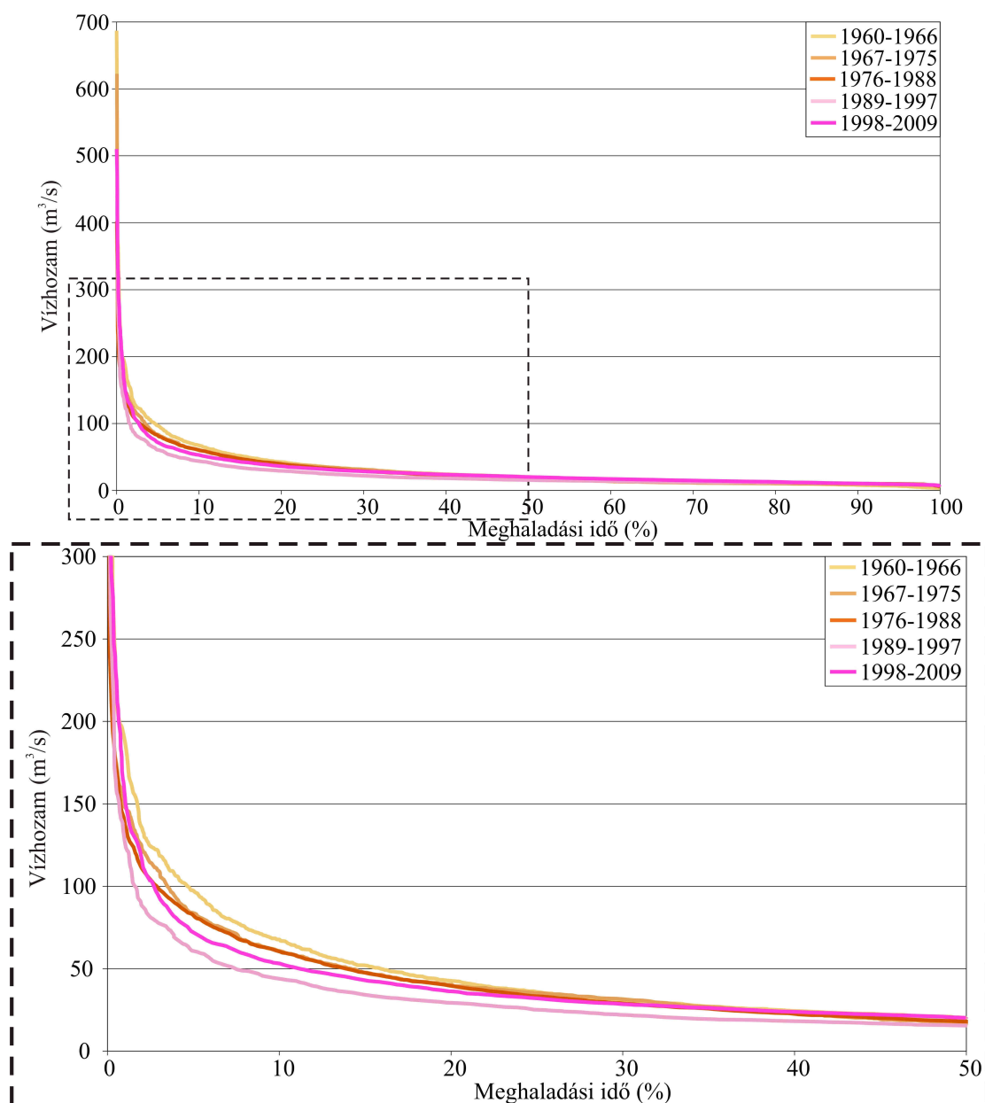
4.4. ábra: A vízhozam-tartósságok (1960-2009) az egyes időszakokban
