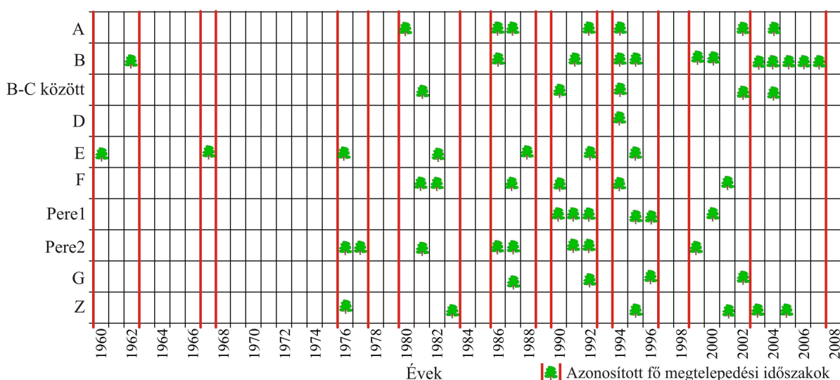
4.36: ábra A vizsgált fák megtelepedési időszakai a kanyarulatokban
