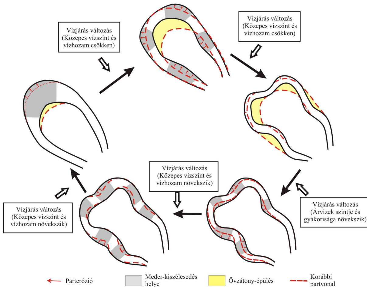
5.1. ábra: A kanyarulatoknak a vízjárás hosszú távú változásához igazodó átalakulásának általános folyamata
