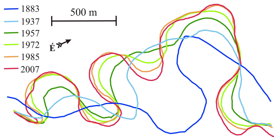
4.22. ábra: A középvonal helyzete az erősen kanyargós (4.) egységen 1883 és 2007 között
