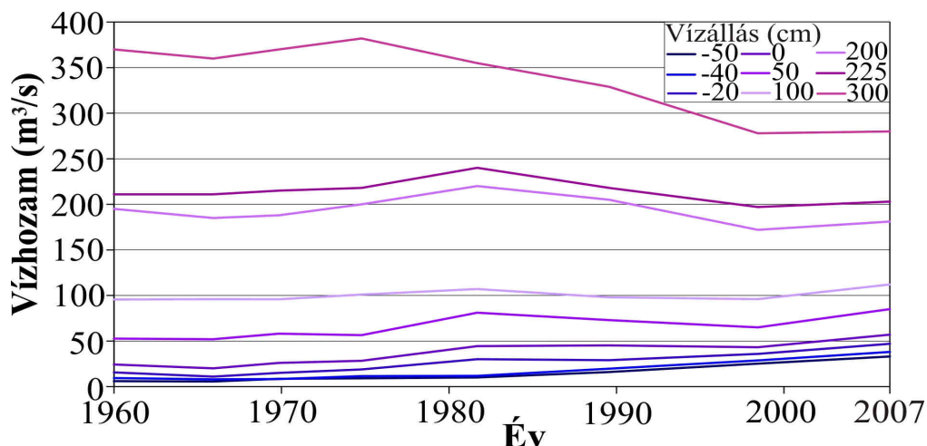
4.8. ábra: Az egyes vízállásokhoz tartozó vízhozamok változása 1960-2007 között
