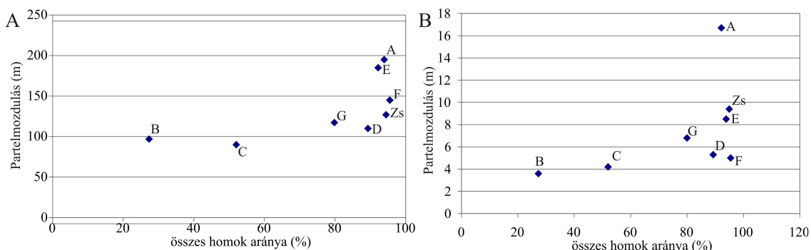
4.32. ábra: A partanyag homoktartalma és a partelmozdulás kapcsolata az 1953-2007 közötti a) és a 2009.08.-2010.08. közötti b) időszakban
