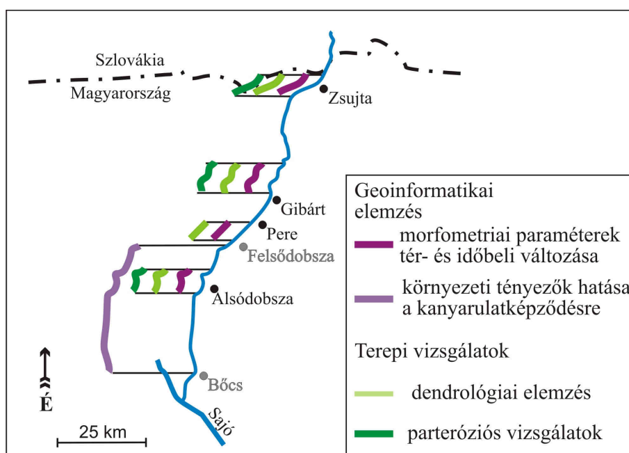
3.3. ábra: A különböző vizsgálatok által érintett Hernád szakaszok
