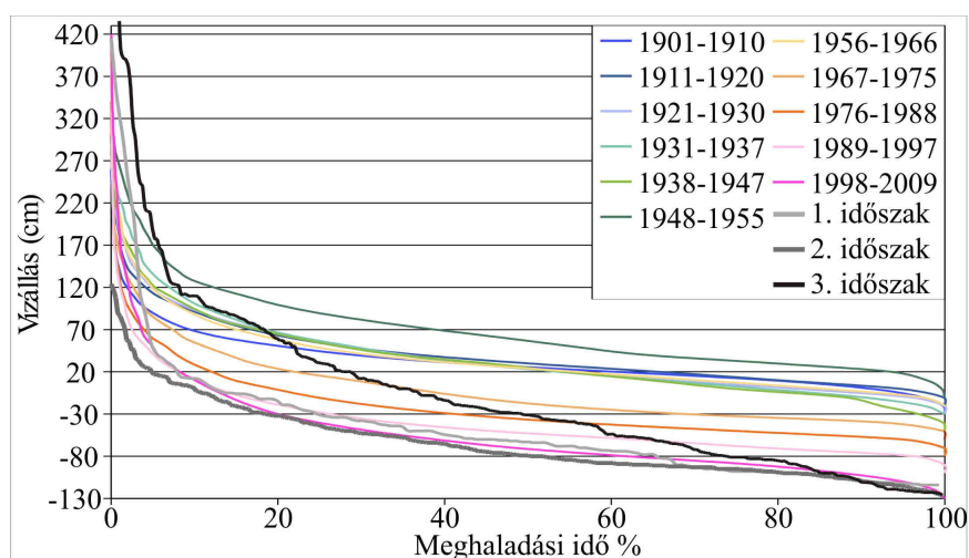
4.29. ábra: Vízállás-tartósság a parteróziós vizsgálat időszakaiban a hidasnémeti vízmércén
