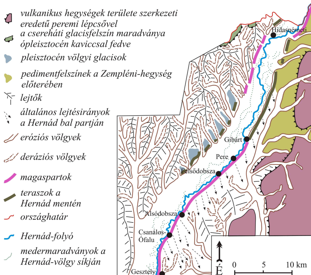
2.3. ábra: A Hernád-völgy geomorfológiai helyzete (Szabó J. 1996)
