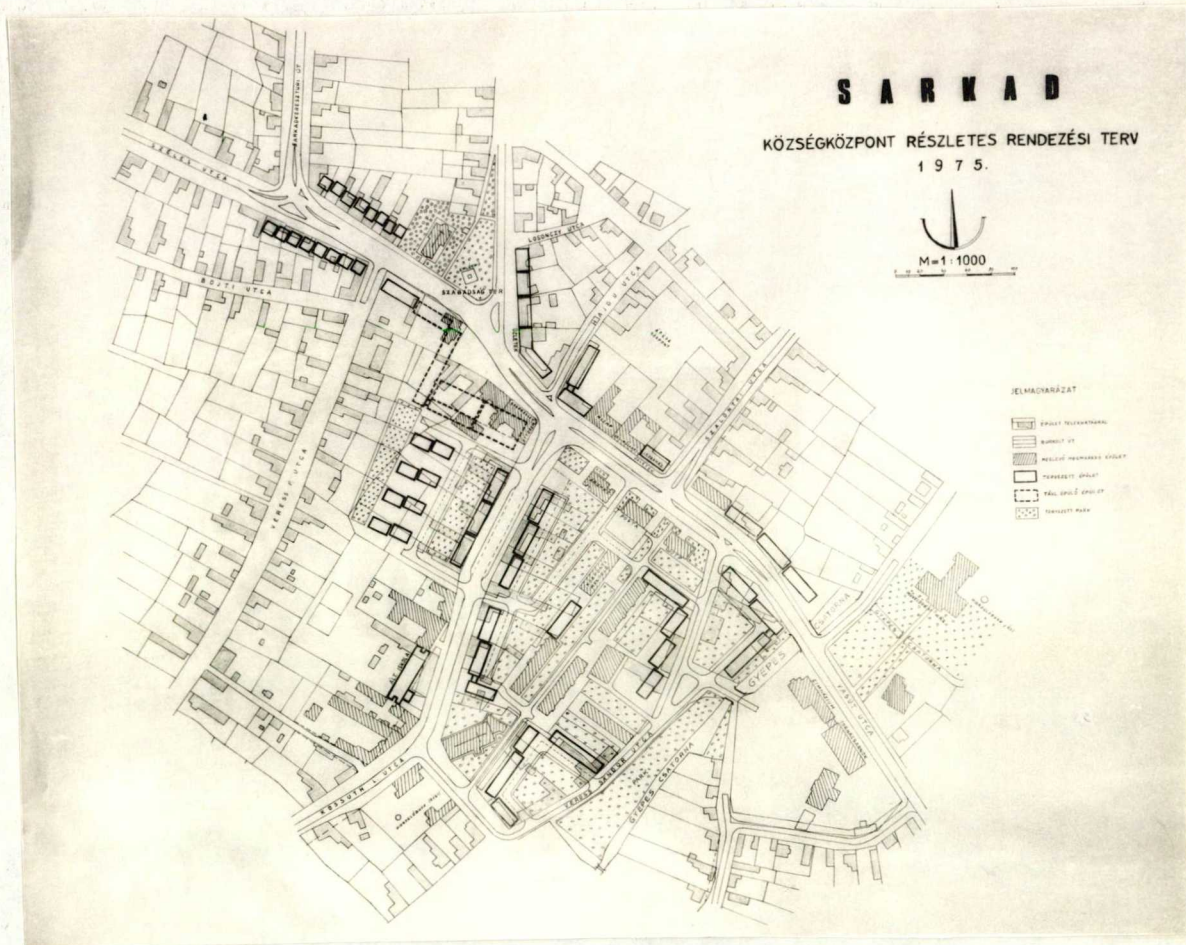
23. ábra Sarkad központjának távlati rendezési terve
