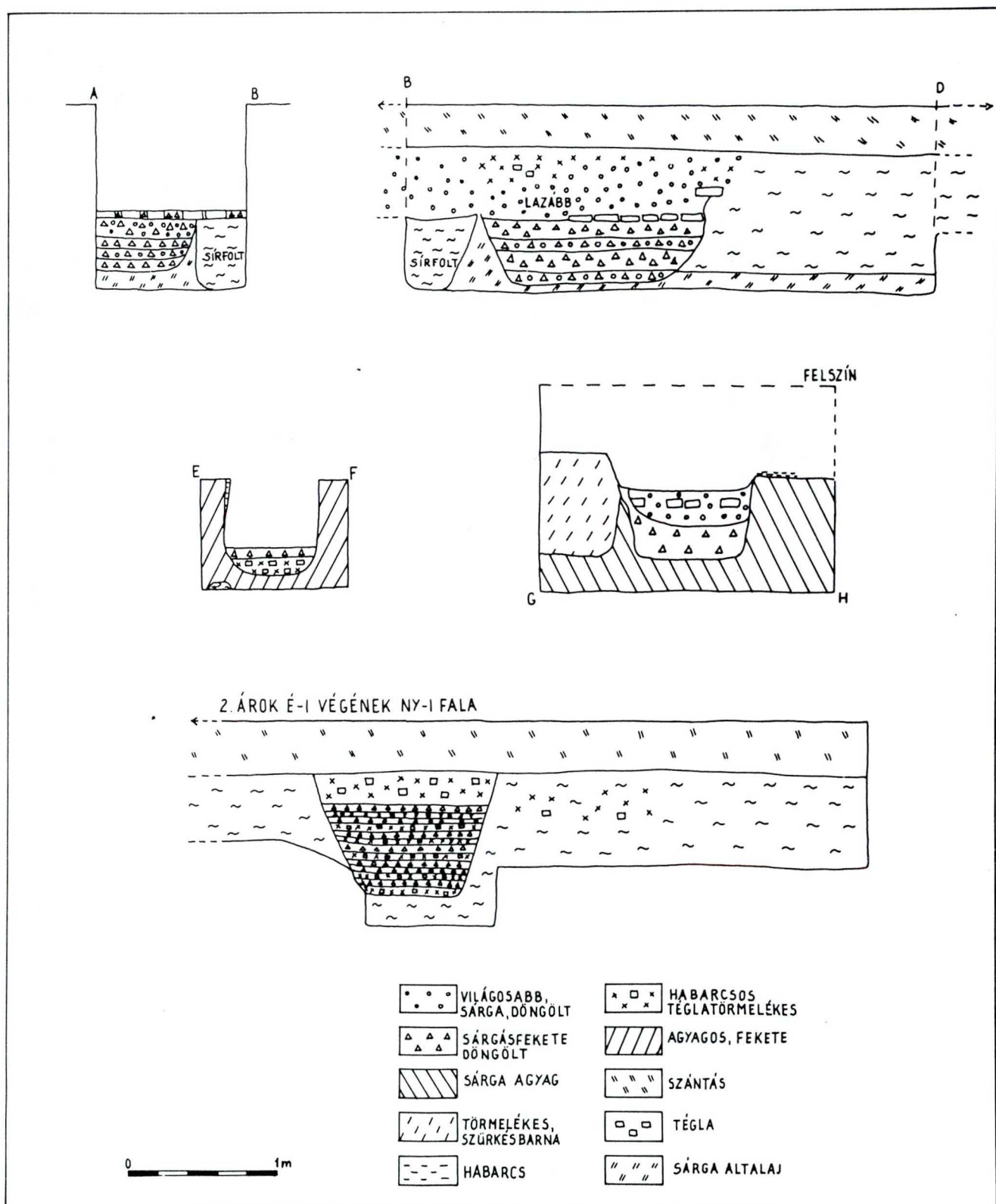
15. kép. Szentbenedek. A templom alapozásának A-B, B-D, E-F, G-H metszete és a 2. árok É-i végének Ny-i fala.
