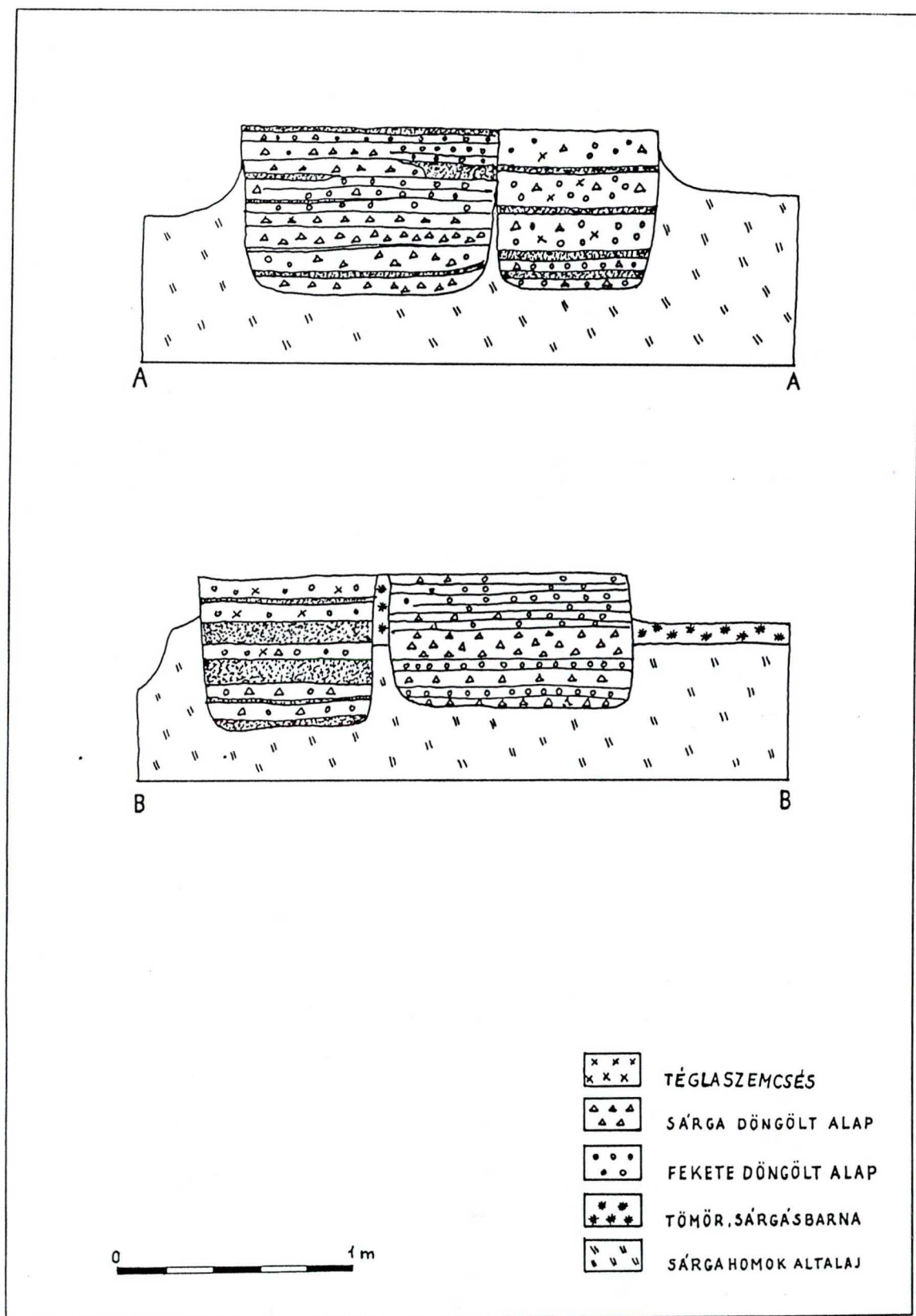
10. kép. Fövenyes. A rotunda és az É-i kör alakú épület alapozásának A-A és B-B metszete.
