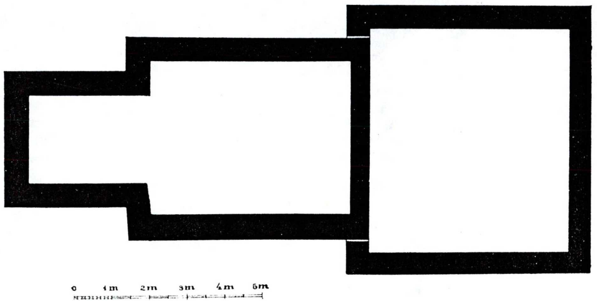
16. kép. Győrke. A templom alaprajza Scherer 1938. 41. nyomán.
