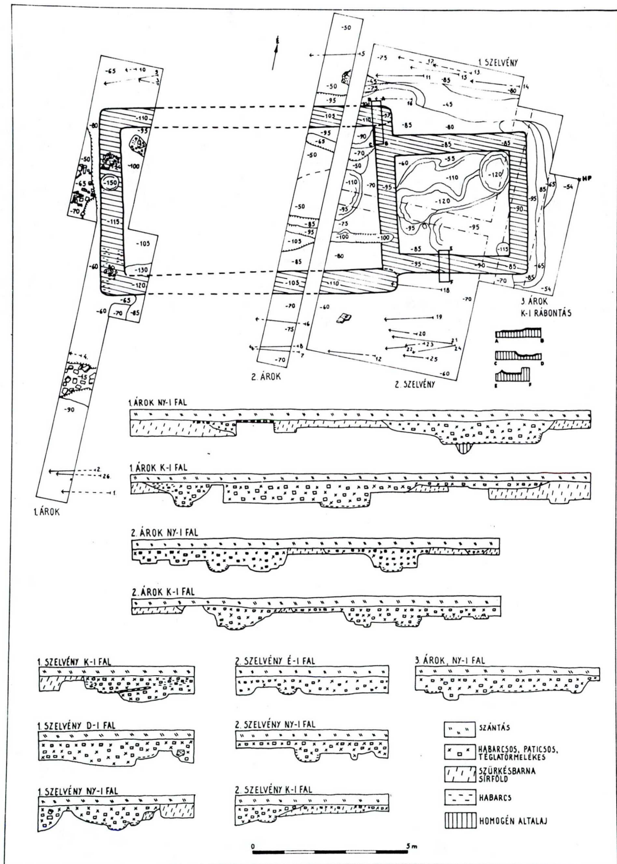
4. kép. Szeregyháza. Az 1986. évi ásatás alaprajza és metszetei.
